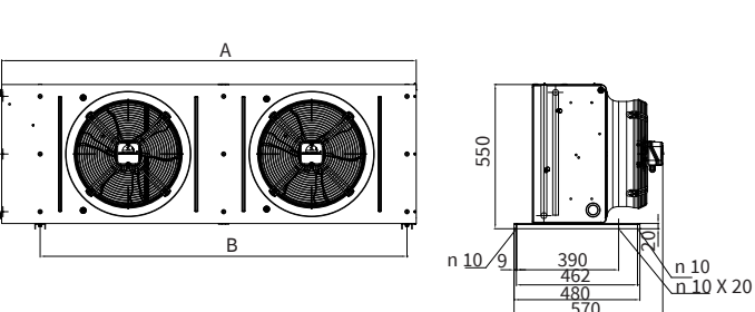
Dimensioni - Dimensions Installazione verticale Vertical installation (V)
