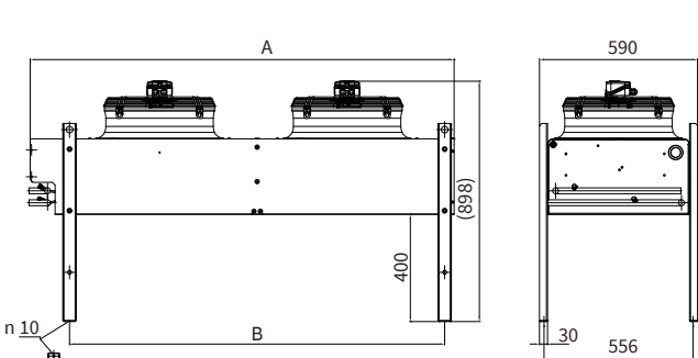
Dimensioni - Dimensions Installazione orizzontale Horizontal installation (H)
